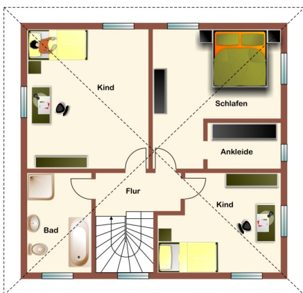
Obergeschoss
